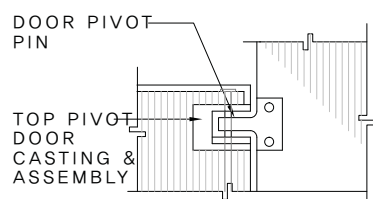
PILASTER / DOOR DETAIL
