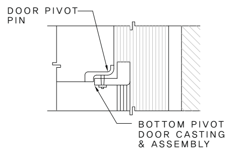
PILASTER / DOOR DETAIL
