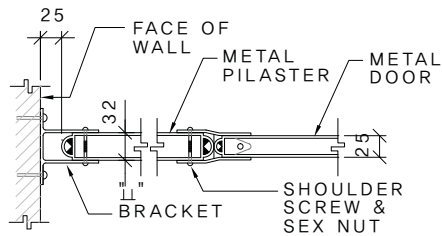
PILASTER / DOOR DETAIL
