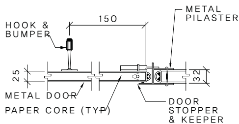
PILASTER / DOOR DETAIL
